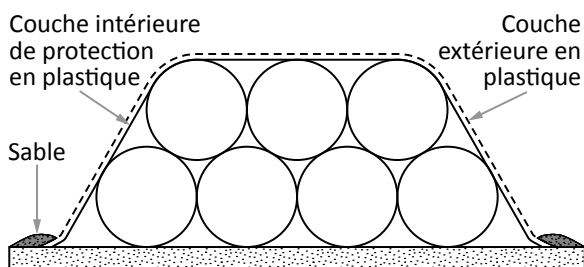
Figure 15-7. Pile de balles rondes d'ensilage (normalement de 3 à 5 balles de longueur).
