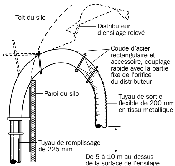
Figure 15-10. Adaptateur suggéré pour la ventilation dans le cas de silos à distributeurs à ailettes.
