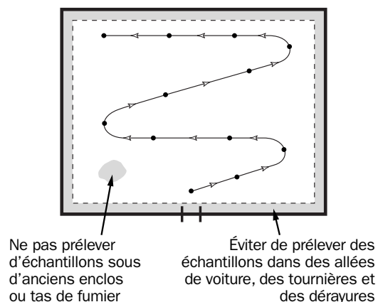
Figure 2-1. Prélèvement d'échantillons-mélanges.
