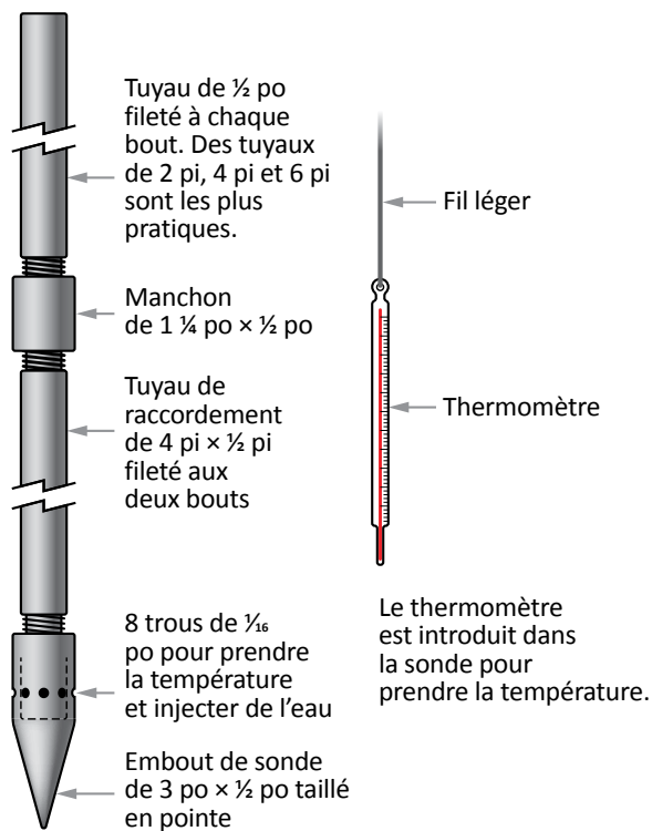
Figure 15-17. Sonde et thermomètre pour le foin.
