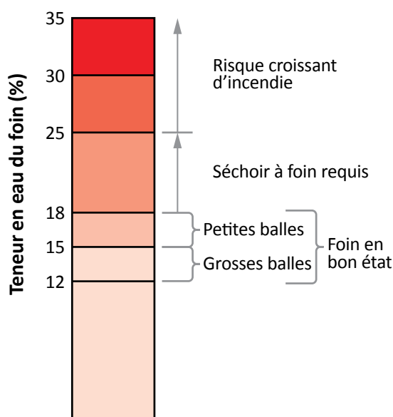
Figure 15-16. Teneur en eau du foin sec.
