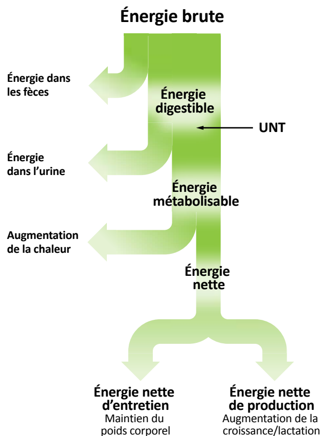
Figure 16-3. Liens entre les différents types d'énergie des aliments.
