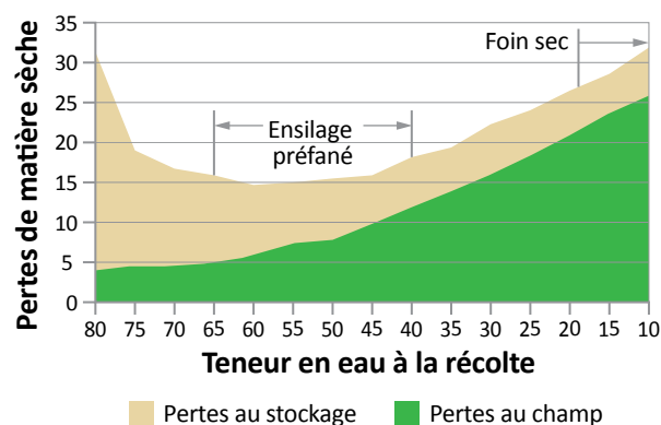
Figure 14-3. Pertes au champ et au stockage.
