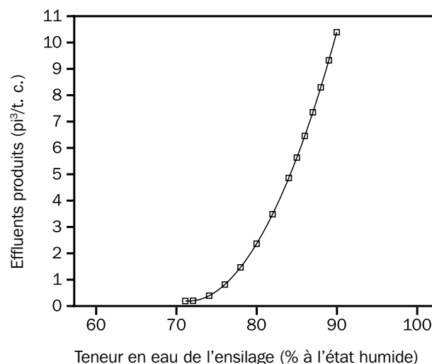
Figure 15-14. Effluents produits dans un silo horizontal selon la teneur en eau de l'ensilage.
