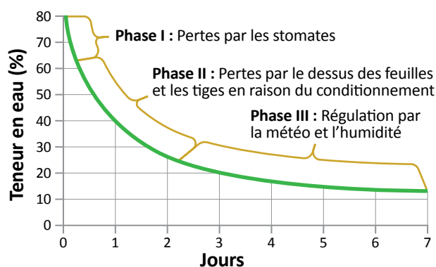
Figure 14-1. Courbe de séchage du foin.
