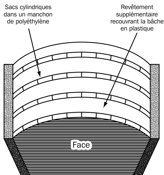
Figure 15-12. Disposition des sacs cylindriques.
