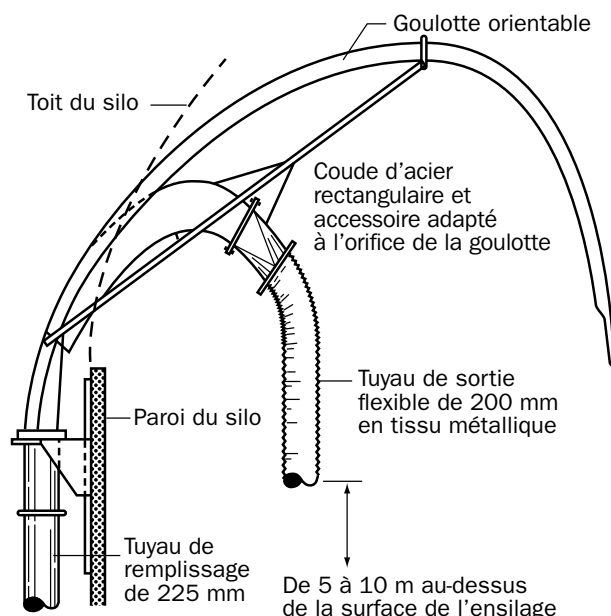
Figure 15-9. Adaptateur suggéré pour la ventilation dans le cas de silos à distributeurs rotatifs.
