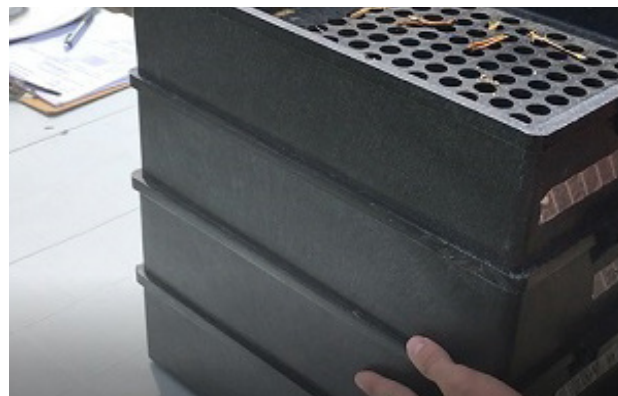
Figure 14-4. Séparateur de particules de l'Université Penn State servant à mesurer la distribution des tailles des particules dans les rations des ruminants.
